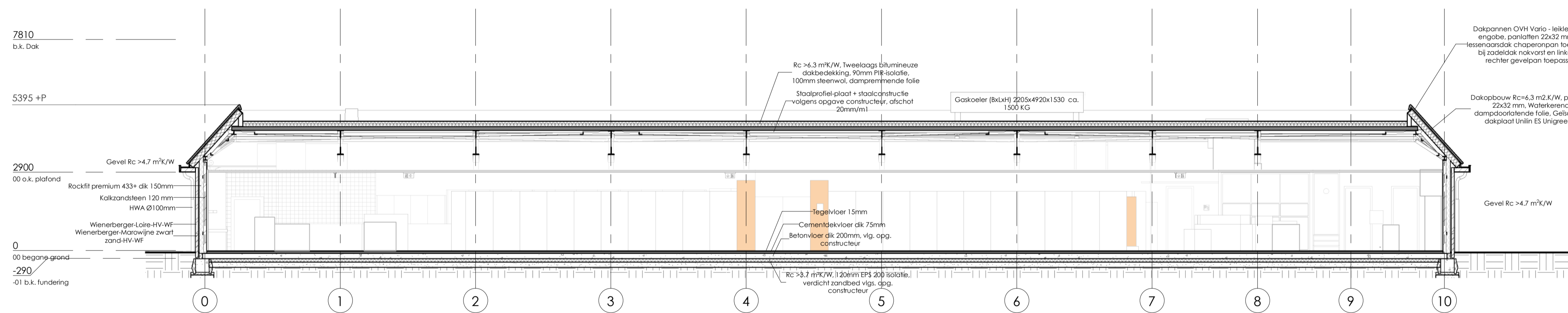
Doorsnede B-B
