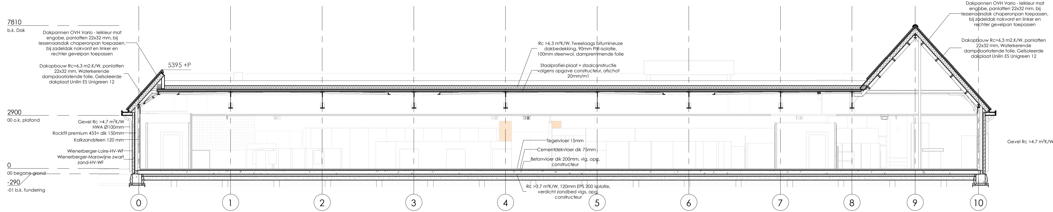
Doorsnede C-C
