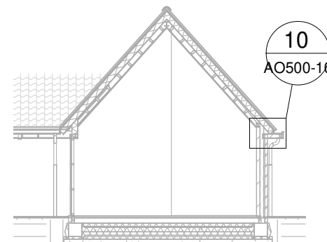
Drsn. I-I
