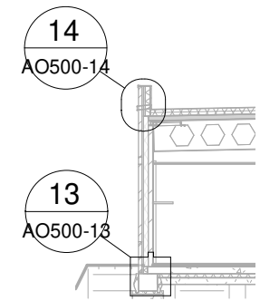
Drsn. M-M
